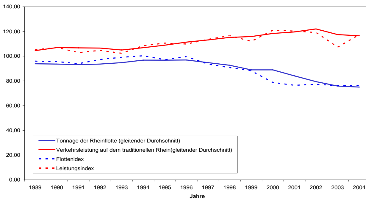
Vergleich zwischen den Entwicklungen der Rheinflotte und der Leistungen auf dem traditionellen Rhein
