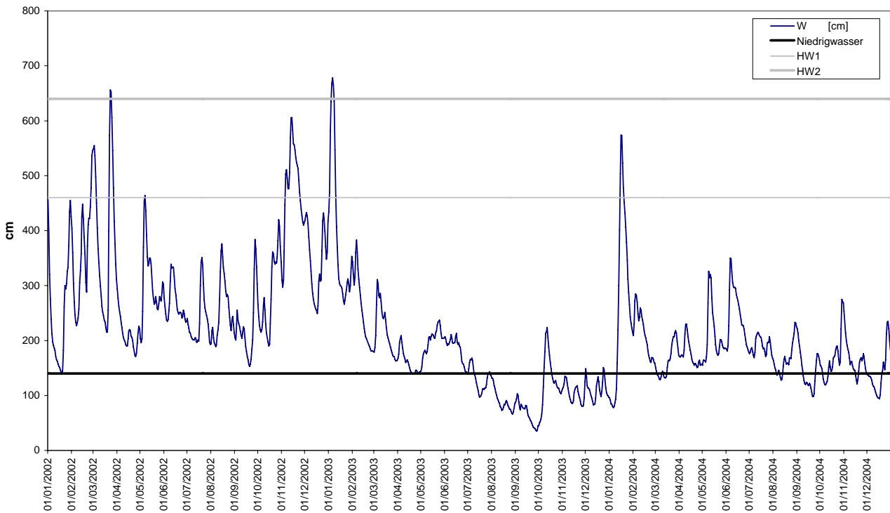
Wasserstände in Kaub in den Jahren 2002,2003 und 2004
