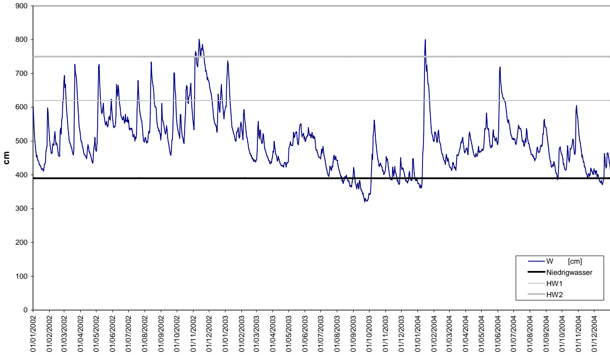
Wasserstände in Maxau in den Jahren 2002, 2003 und 2004
